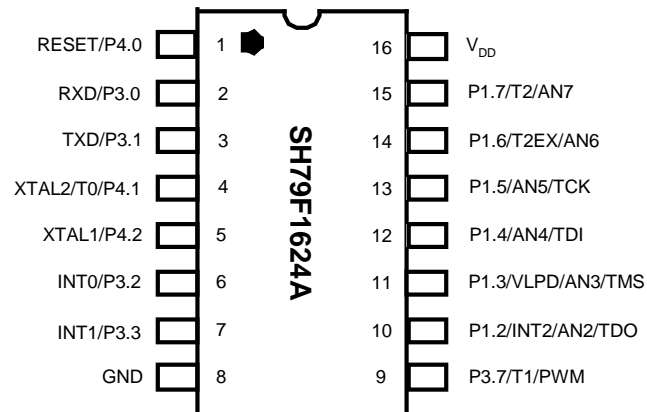
引脚配置图
